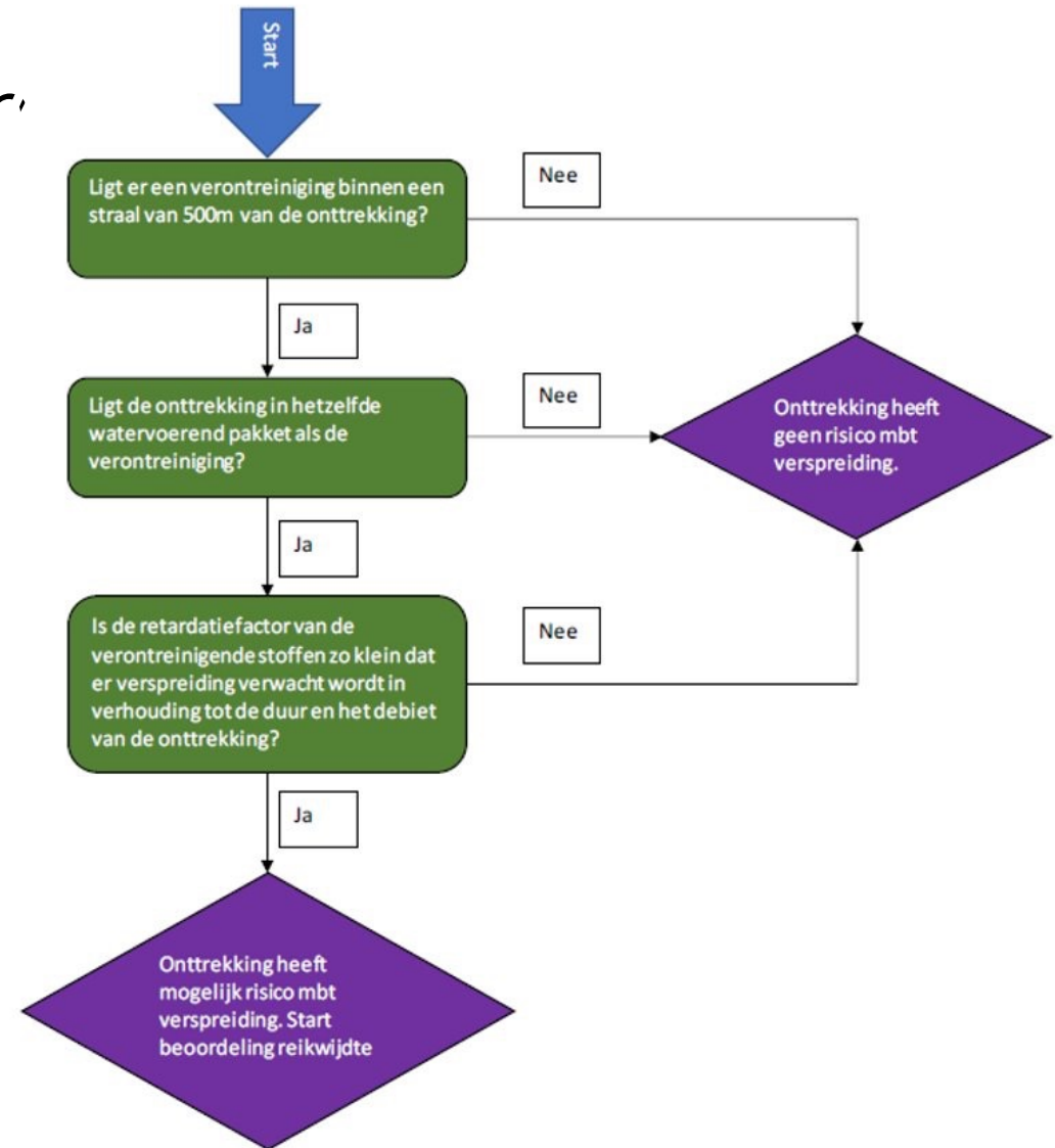
Figuur 1: stroomschema vragen eerste stap beoordeling grondwateronttrekking
